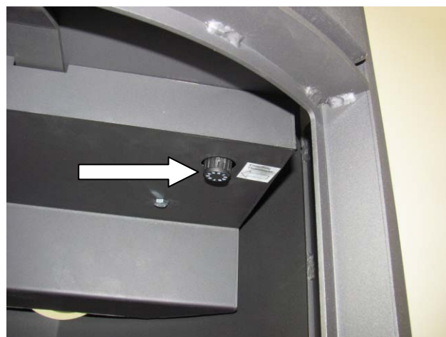
Fig. 13 : molette de réglage du thermorégulateur
