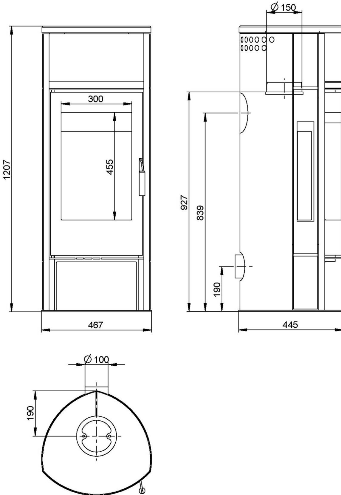
Fig. 1 : plan coté Lucky K100A
