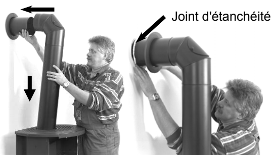
Fig. 5 : montage du tuyau de fumée
