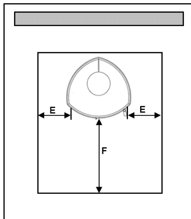
Fig. 4 : protection anti-étincelles K100A
