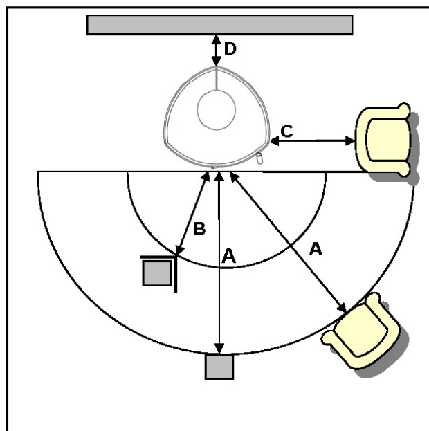
Fig. 3 : distances de sécurité K100A
