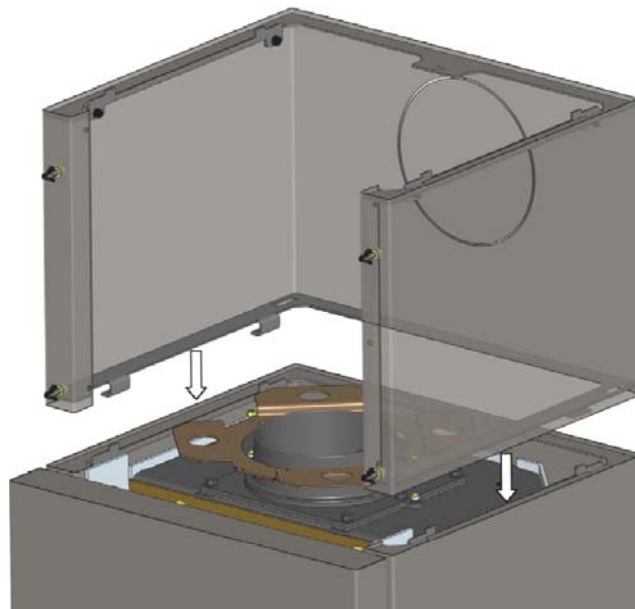
Fig. 14 : montage du module accumulateur de chaleur
