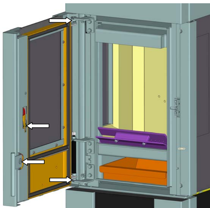
Fig. 40 : mécanisme de la porte
