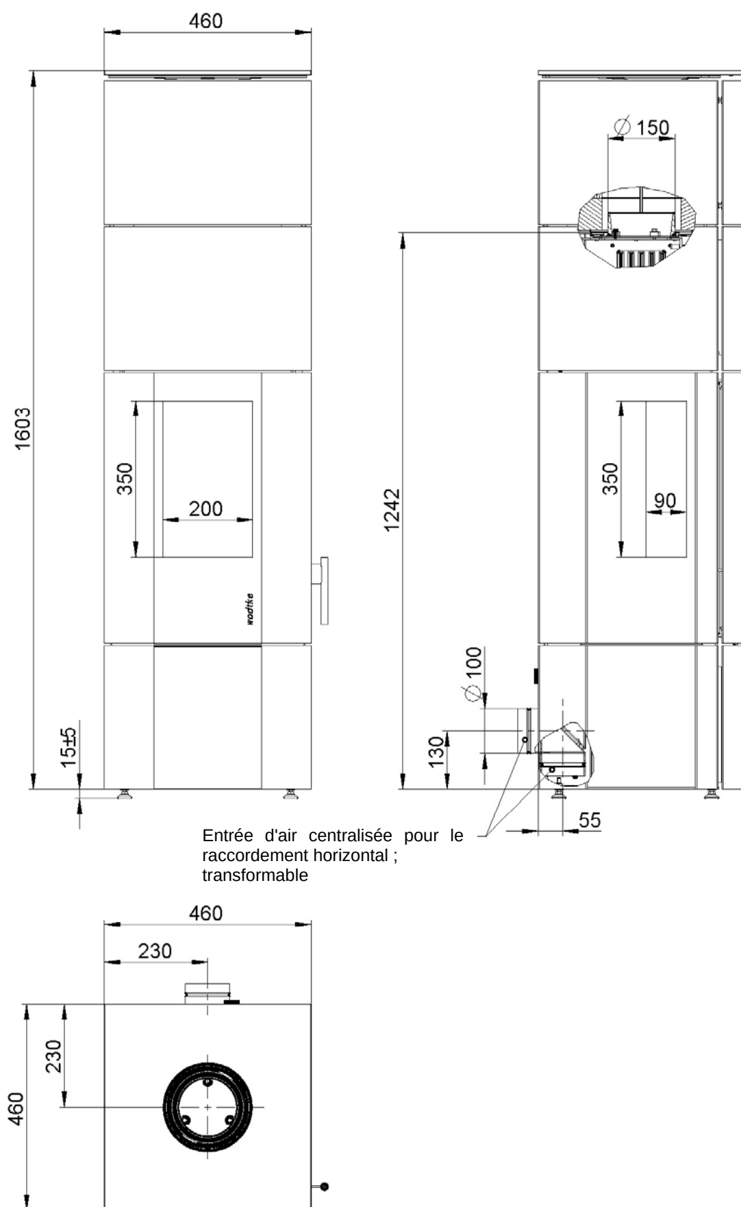
Fig. 2 : plan coté KK 61-1
