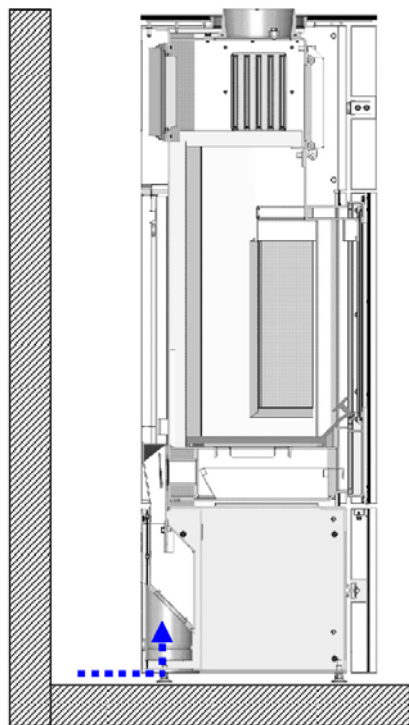
Fig. 21 : aspiration depuis la pièce d'installation
