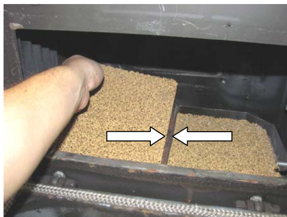
Fig. 10 : introduction du HiClean-Filter®
