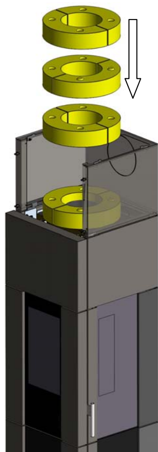
Fig. 16 : mise en place des pierres accumultrices wotke
