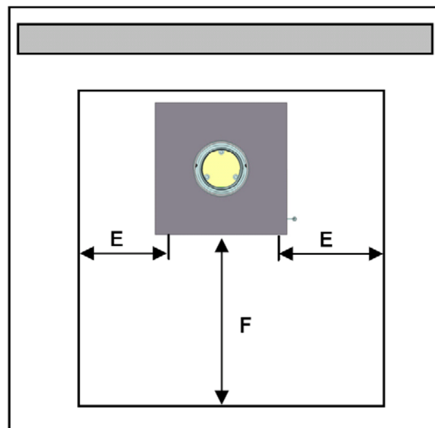
Fig. 6 : protection anti-étincelles KK 61
