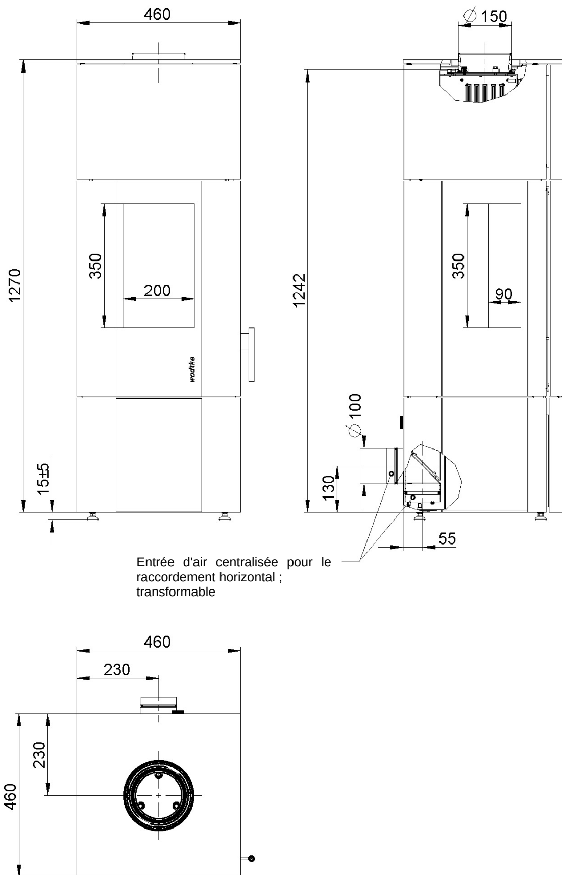
Fig. 1 : plan coté KK 61
