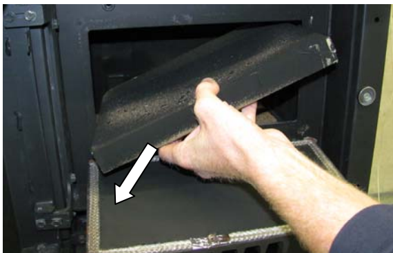
Fig. 9 : retrait du déflecteur supérieur
