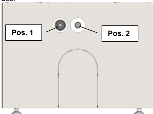
Fig. 36 : position du thermorégulateur et du régulateur d'air secondaire
