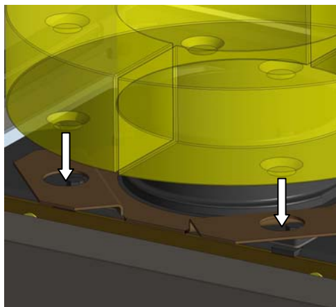
Fig. 17 : détail du tenon de positionnement
