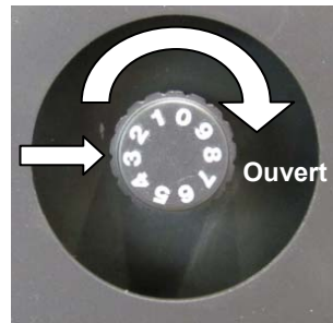
Fig. 38 : réglage thermorégulateur
