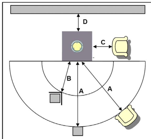
Fig. 5 : distances de sécurité KK 61
