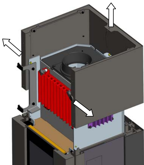
Fig. 28 : démontage de l'habillage supérieur
