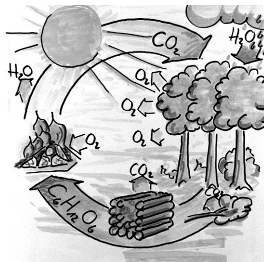
Fig. 34 : cycle du CO 2
