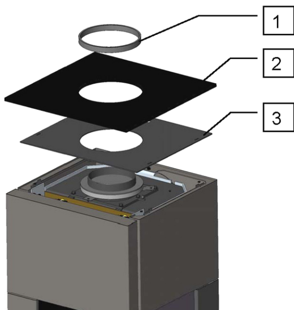
Fig. 12 : retrait du couvercle supérieur
