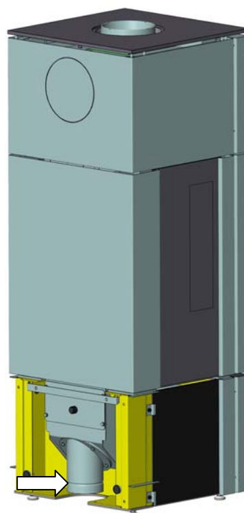
Fig. 19 : manchon d'air de combustion centralisé
