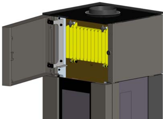
Fig. 7 : ouverture du volet supérieur
