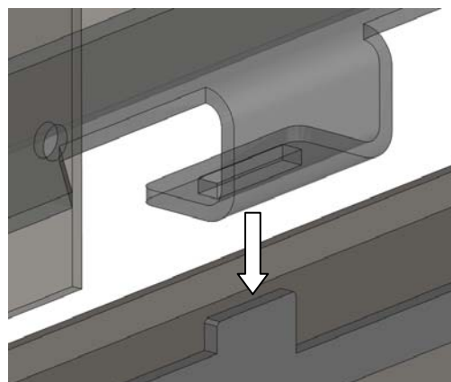
Fig. 15 : détail du montage du module accumulateur de chaleur
