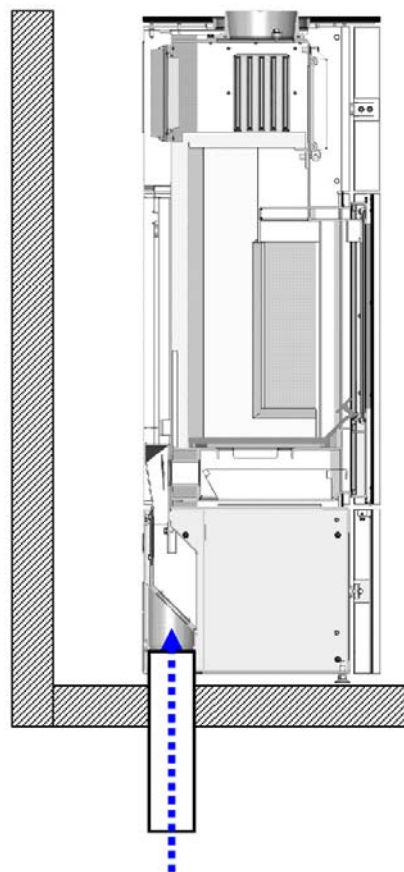
Fig. 22 : depuis en bas cave / sous-sol (recommandation)
