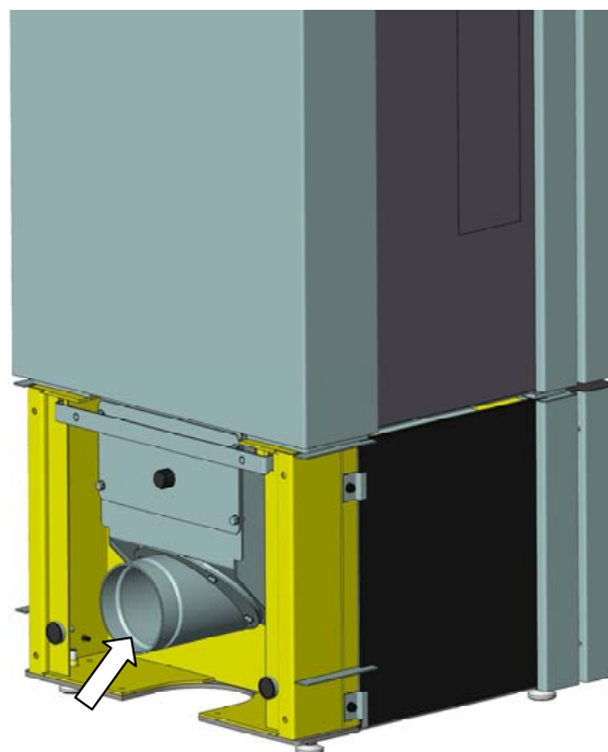
Fig. 20 : manchon d'air de combustion horizontal
