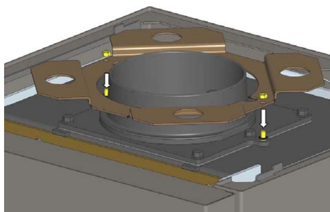
Fig. 13 : montage du support combiné
