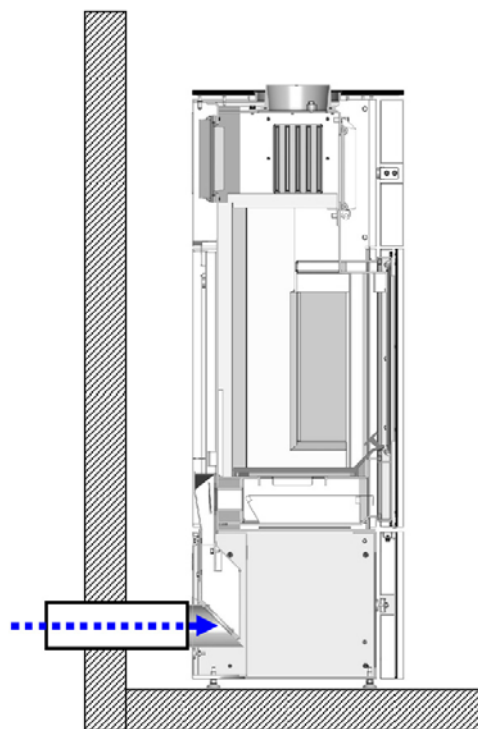
Fig. 23 : depuis la pièce adjacente ou par un conduit d'air séparé
