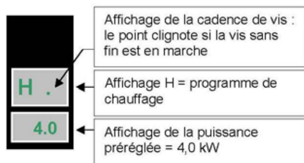
Fig. 7 : panneau de commande mode de chauffage
