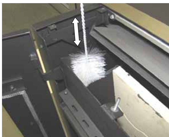
Fig. 41 : nettoyage du tirage de gaz de combustion
