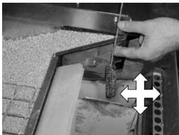
Fig. 69 : nettoyage du tirage de gaz de combustion inférieur
