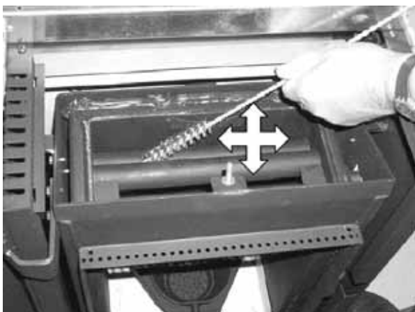
Fig. 122 : nettoyage de l'échangeur thermique à eau
