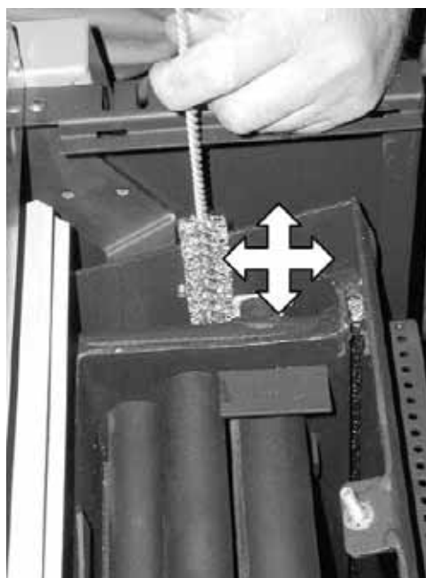
Fig. 136 : nettoyage des tirages de gaz de combustion
