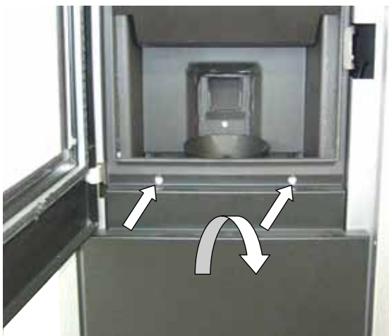
Fig. 153 : démontage de l'habillage avant
