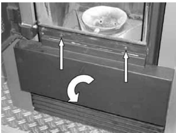
Fig. 123 : démontage de l'habillage de la trappe de visite
