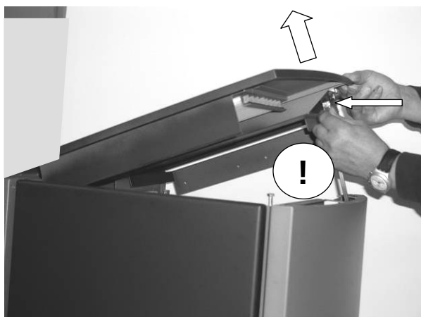
Fig. 146 : desserrage du câble du panneau de commande
