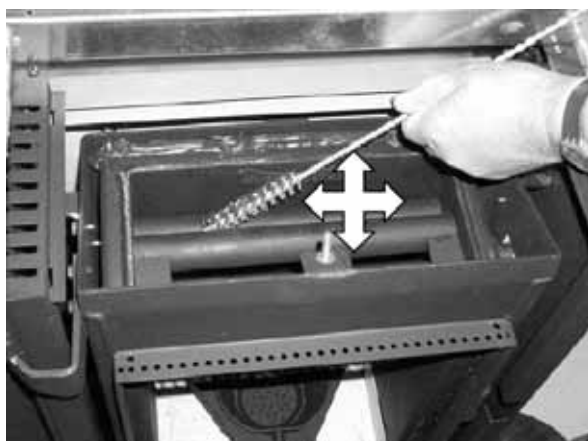
Fig. 137 : nettoyage de l'échangeur thermique à eau
