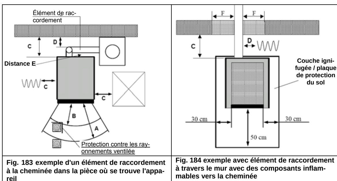
Figures d'explication des distances de prévention des incendies
