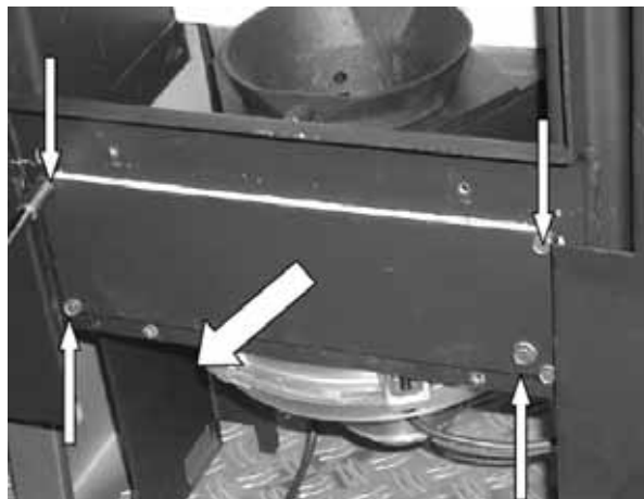
Fig. 58 : démontage du couvercle de révision
