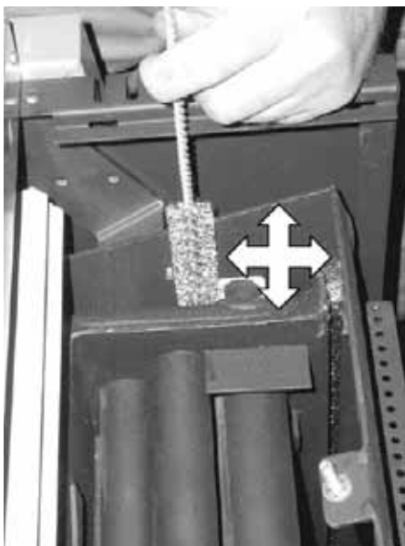
Fig. 121 : nettoyage des tirages de gaz de combustion
