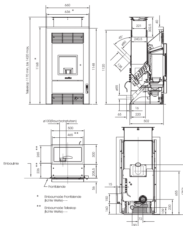
Fig. 187 : plan coté "PE SX"
