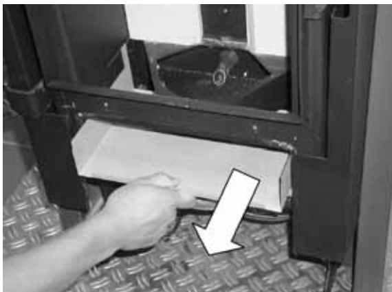
Fig. 157 : retrait de la tôle de fond
