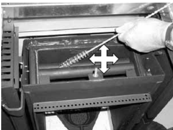
Fig. 152 : nettoyage de l'échangeur thermique à eau
