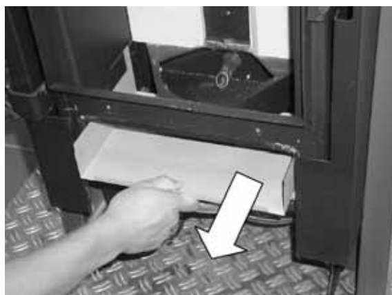
Fig. 170 : retrait de la tôle de fond
