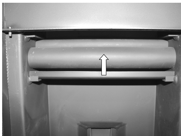
Fig. 164 : démontage du déflecteur inférieur
