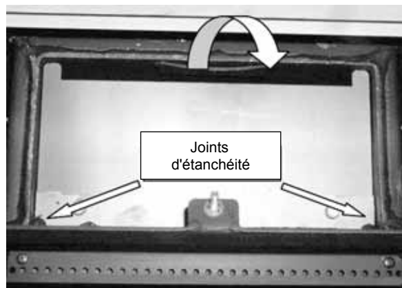
Fig. 148 : démontage du déflecteur supérieur
