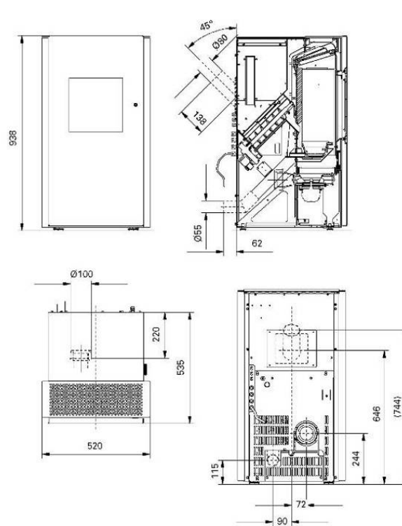
Fig. 189 : plan coté "Frank SX"
