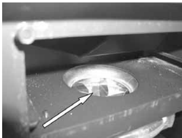
Fig. 91 : soufflerie des gaz de fumée
