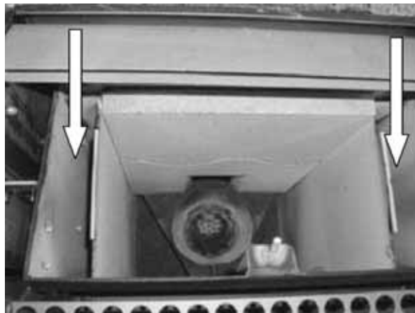
Fig. 68 : nettoyage des tirages de gaz de combustion
