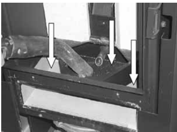
Fig. 60 : nettoyage du support du pot
