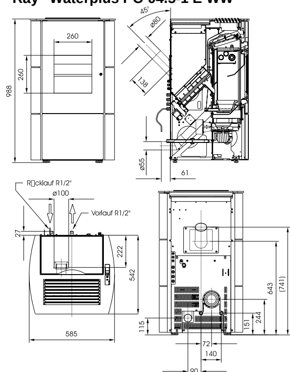
Fig. 192 : plan coté "Ray" Waterplus
