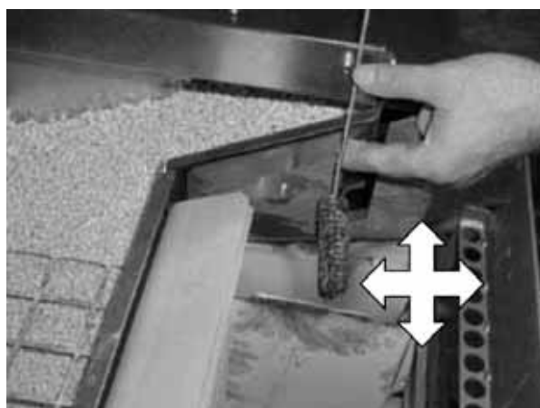
Fig. 83 : nettoyage du tirage des gaz de combustion
