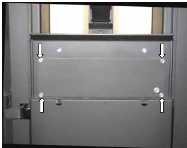
Fig. 43 : démontage du couvercle de révision
