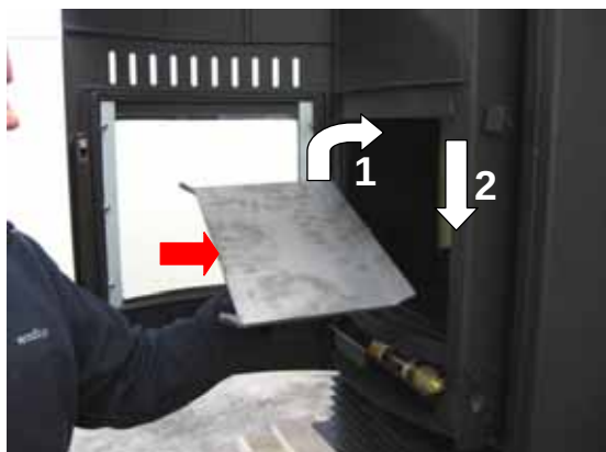
Fig. 105 : retrait du déflecteur avant
