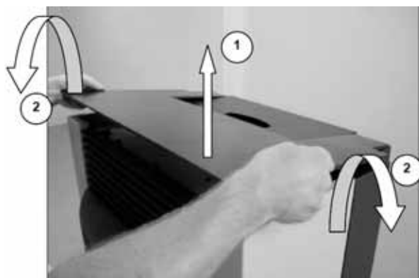
Fig. 106 : démontage des habillages
