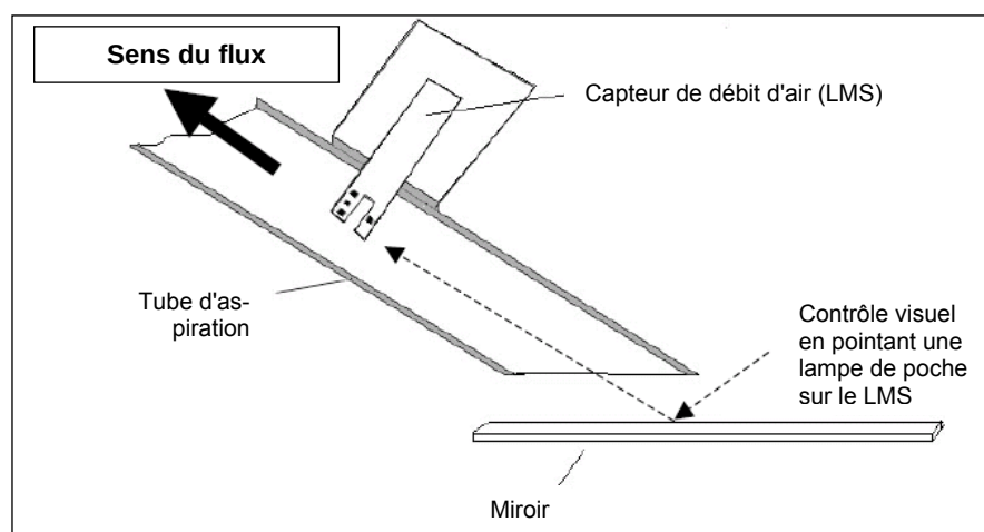
Fig. 178 : croquis de fonctionnement capteur de débit d'air
