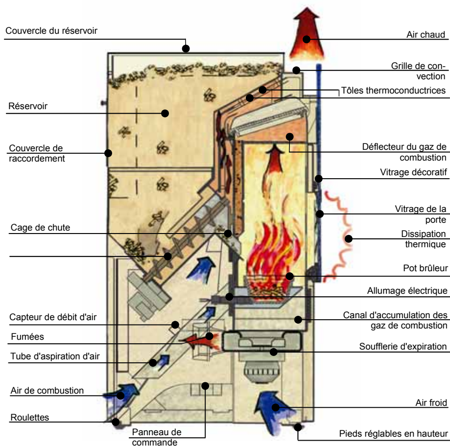
Fig. 3 : croquis de fonctionnement poêle à pellets Airplus
