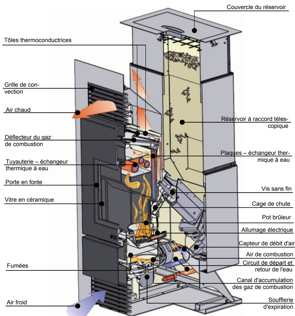
Fig. 4 : croquis de fonctionnement PE Waterplus
