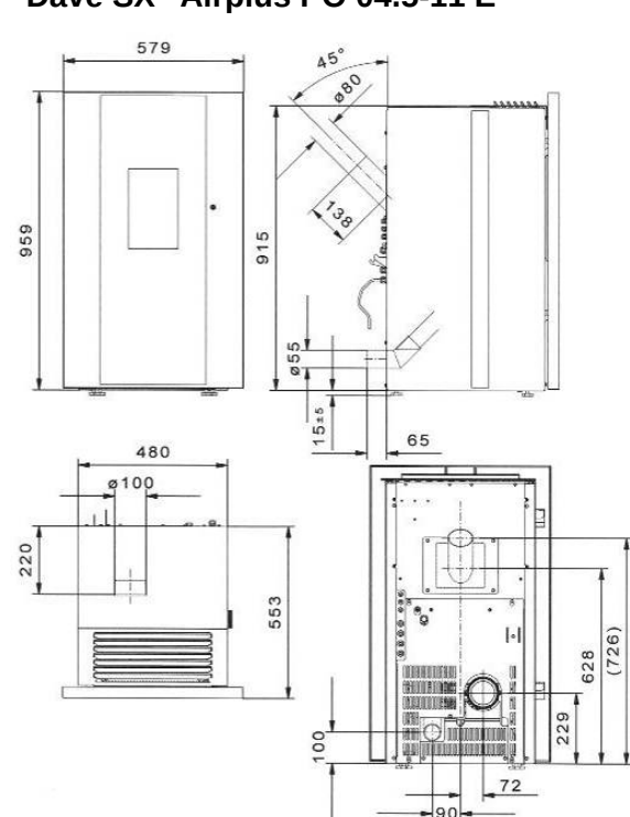
Fig. 193 : plan coté "Dave SX"
