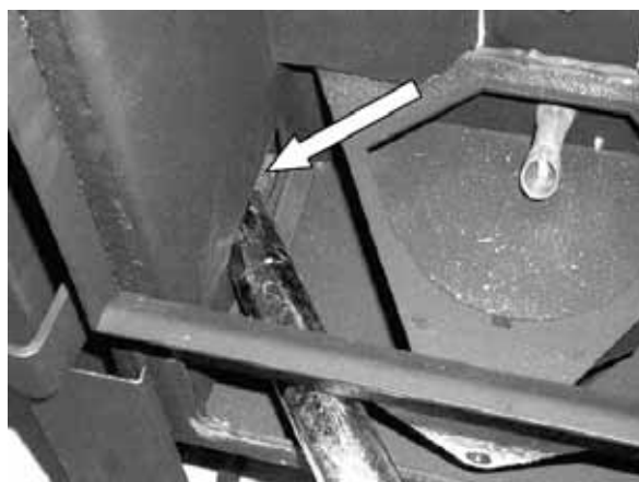
Fig. 90 : nettoyage des tirages de gaz de combustion inférieurs
