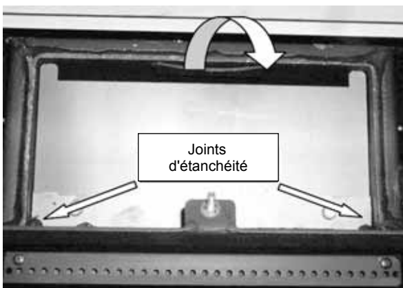
Fig. 162 : retrait du déflecteur supérieur
