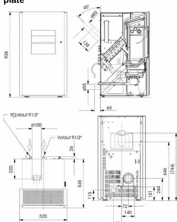
Fig. 190 : plan coté "Frank" Waterplus
