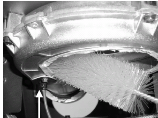
Fig. 176 : position du capteur des gaz de fumée
