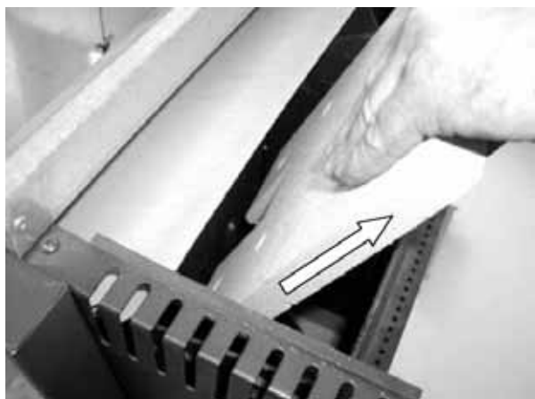
Fig. 56 : retrait de la chamotte
