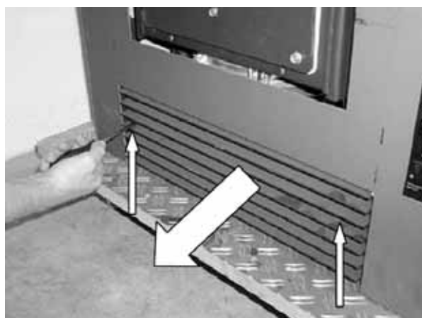
Fig. 130 : démontage du tablier d'habillage
