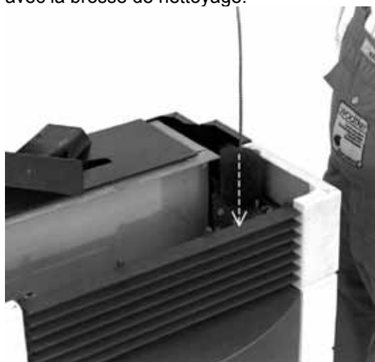
Fig. 109 : nettoyage des tirages de gaz de combustion
