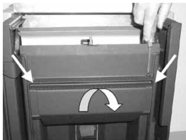
Fig. 119 : démontage de la tôle de déflexion
