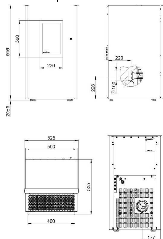
Fig. 186 : plan coté "Pat SX"
