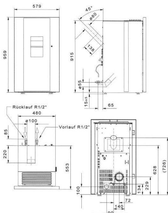
Fig. 194 : plan coté "Dave" Waterplus
