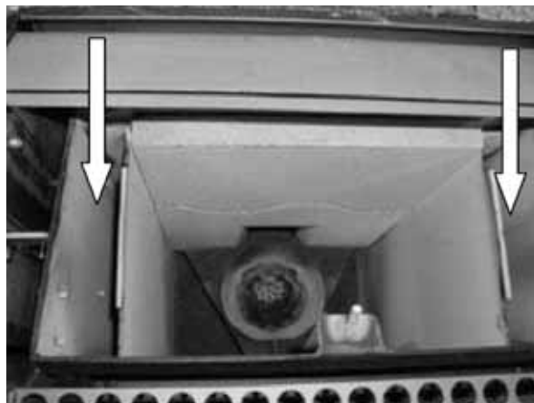
Fig. 54 nettoyage des tirages de gaz de combustion
