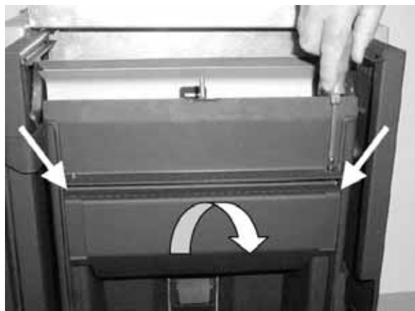
Fig. 134 : démontage de la tôle de déflexion
