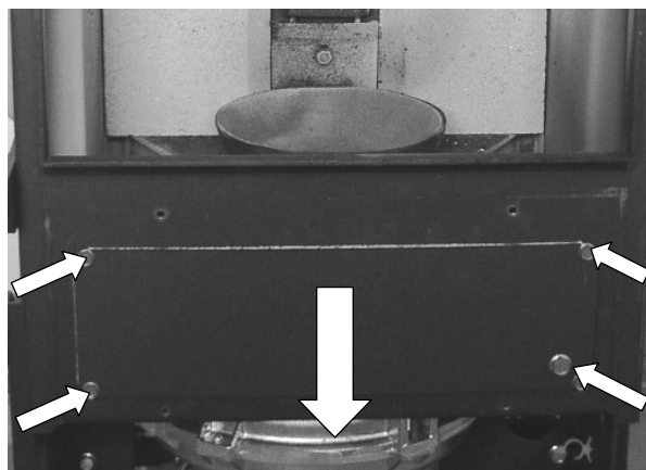
Fig. 86 : démontage du couvercle de révision
