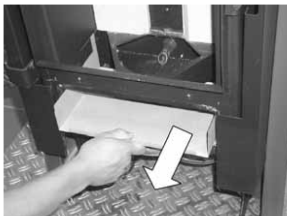
Fig. 141 : retrait de la tôle de fond
