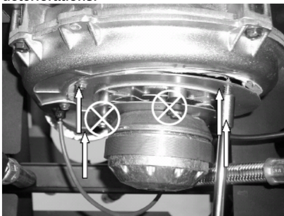
Fig. 174 : démontage du moteur de la soufflerie
