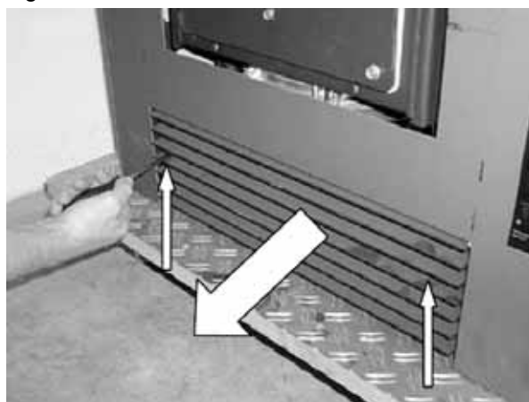
Fig. 64 : démontage du tablier d'habillage
