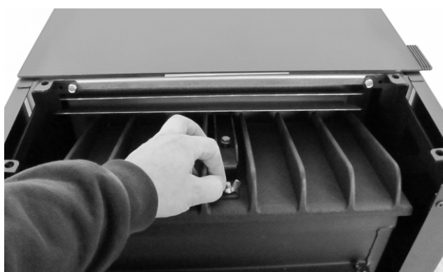
Fig. 93 : démontage du couvercle en fonte
