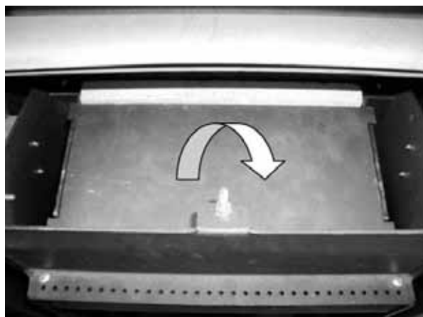
Fig. 81 : retrait du déflecteur supérieur
