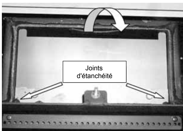
Fig. 133 : retrait du déflecteur supérieur
