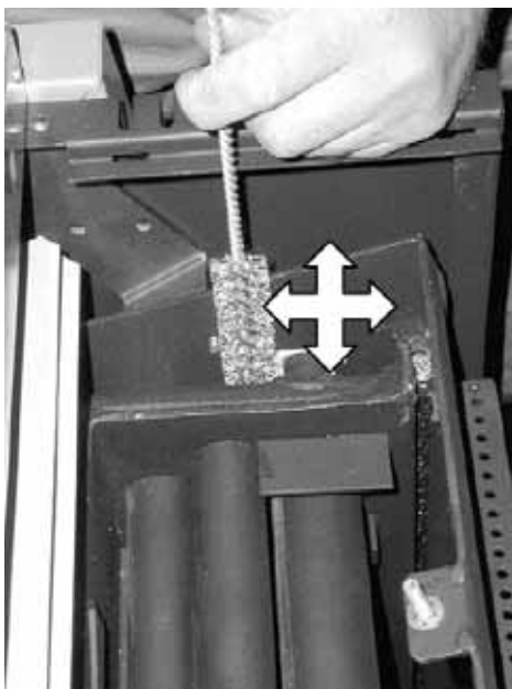
Fig. 151 : nettoyage des tirages de gaz de combustion
