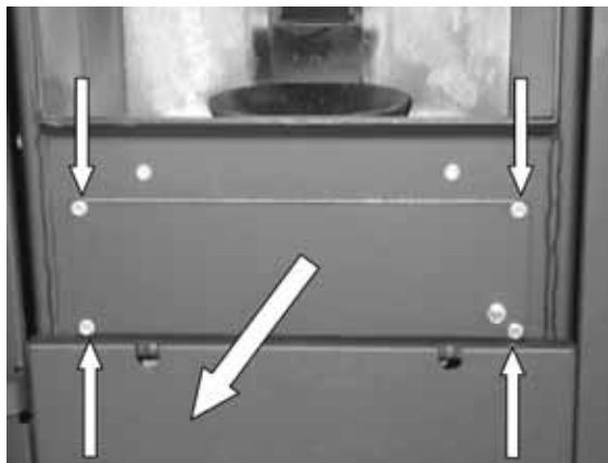
Fig. 71 : démontage du couvercle de révision
