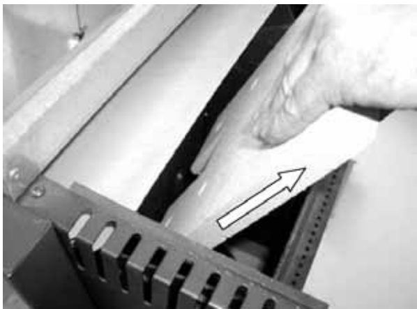
Fig. 84 : retrait de la chamotte
