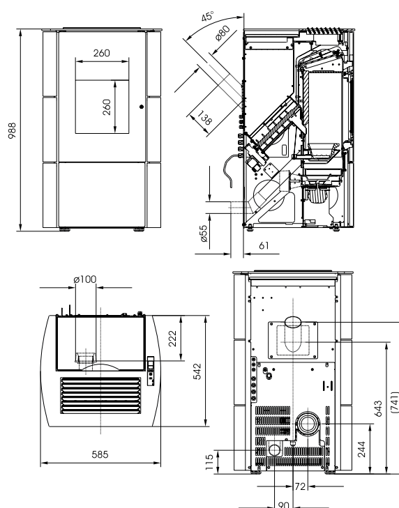
Fig. 191 : plan coté "Ray SX"
