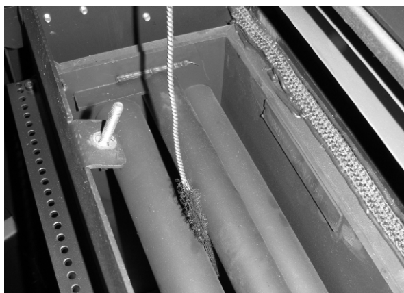
Fig. 166 : nettoyage de l'échangeur thermique à eau
