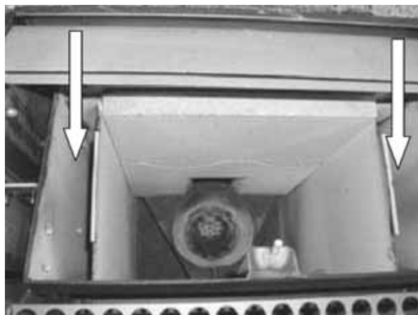
Fig. 82 : nettoyage des tirages des gaz de combustion
