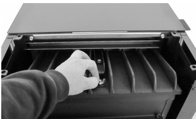
Fig. 161 : démontage du couvercle en fonte
