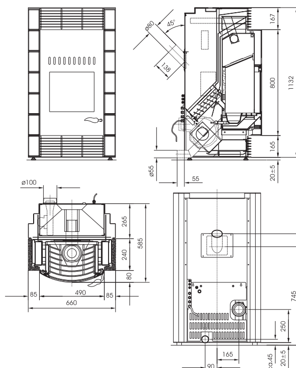
Fig. 195 : plan coté "Topline" Airplus
