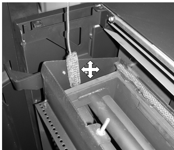
Fig. 165 : nettoyage des tirages de gaz de combustion
