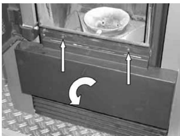
Fig. 57 : démontage de l'habillage de la trappe de visite
