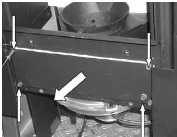
Fig. 124 : démontage du couvercle de révision
