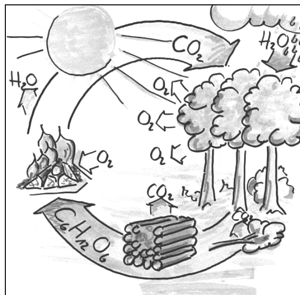
Fig. 185 : Le cycle du CO 2
