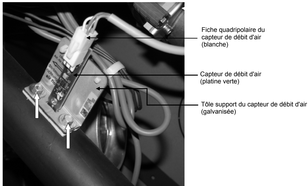
Fig. 182 : capteur de débit d'air
