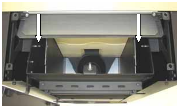
Fig. 40 : nettoyage des tirages de gaz de combustion
