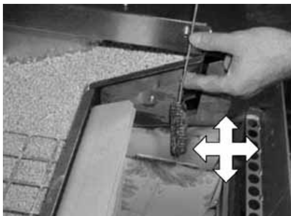
Fig. 55 : nettoyage du tirage de gaz de combustion
