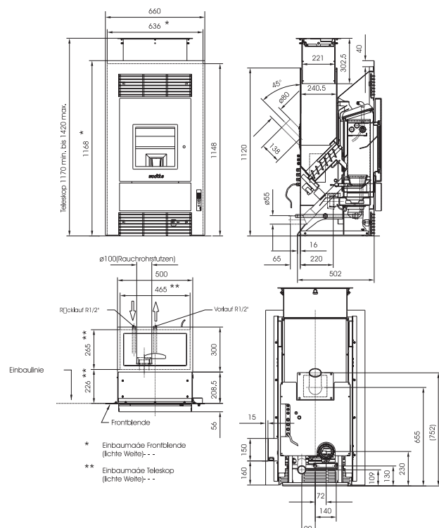
Fig. 188 : plan coté "PE" Waterplus
