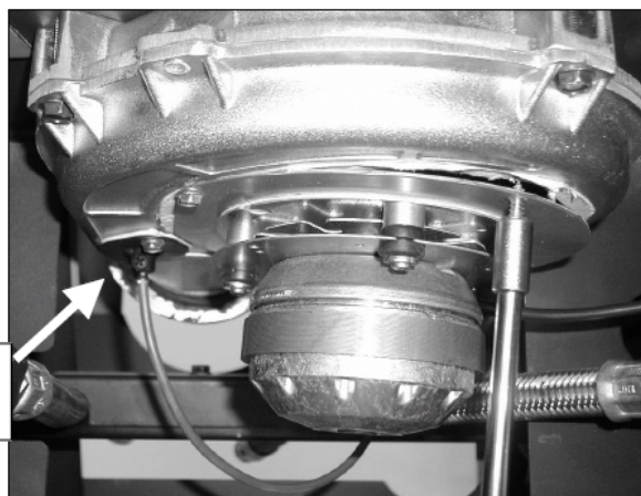
Douille immergée de la soufflerie des fumées
