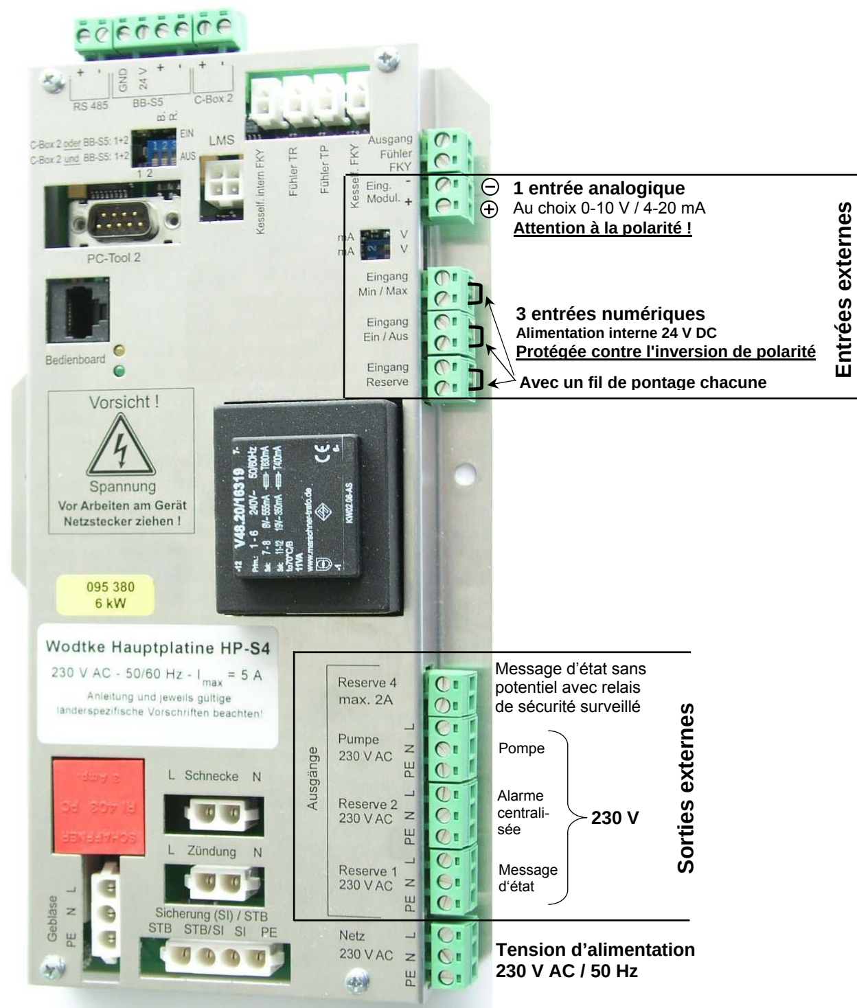
Carte-mère principale avec connecteurs de raccordement pour régulateurs externes
