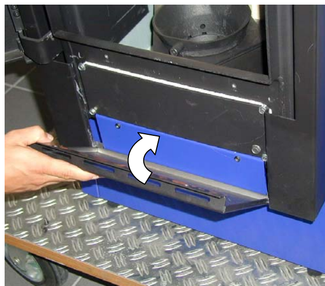
Fig. 8 : Remontez l'habillage de l'ouverture de révision dans le sens inverse du démontage, en vous reportant à la description donnée aux figures de 3 à 5, fixez-le à l'aide des deux vis.
